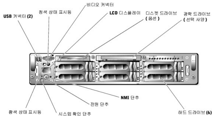
그림 1-1. 전면 패널 구조 및 표시등
