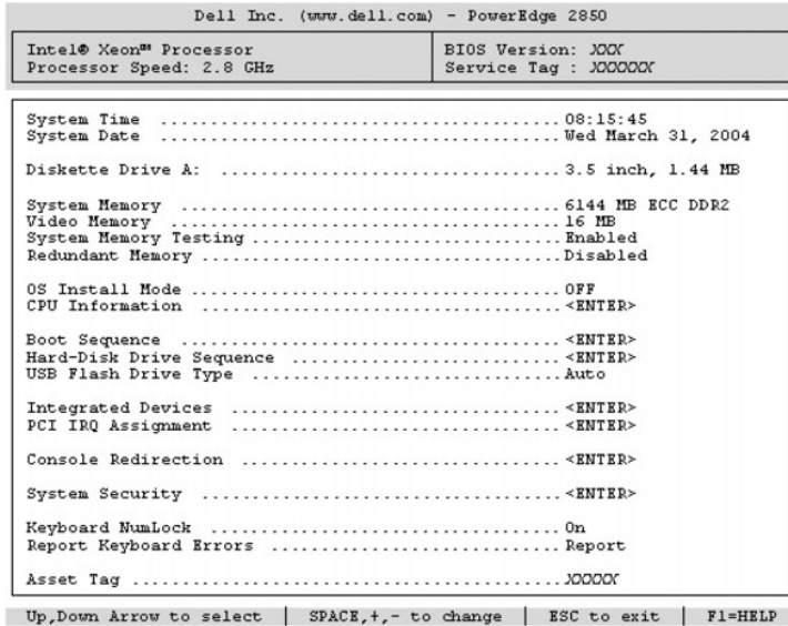
그림 3-1. 시스템 설치 프로그램 기본 화면
