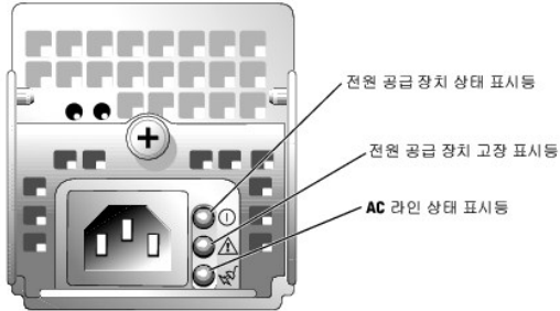
그림 1-4. 중복 전원 공급 장치 표시등
