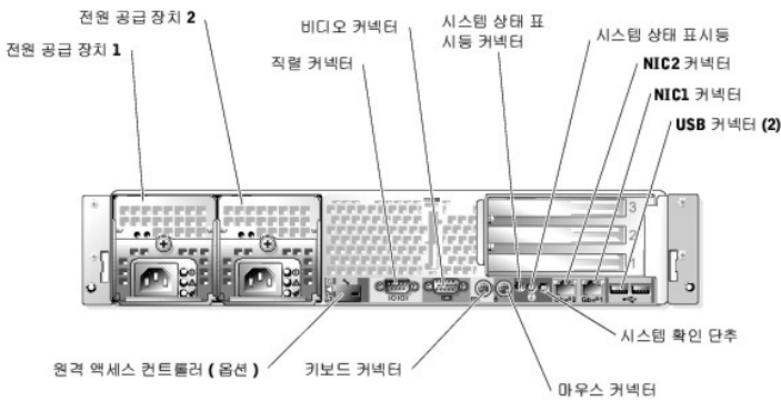
그림 1-3. 후면 패널 구조 및 표시등
